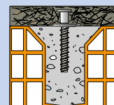
Solaio esistente con o senza caldana
