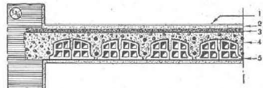
Fig. 43 — SOLAIO "MIOZZO SALERNI", - 1 Pavimento - 2 Lastre isolanti - 3 Sottofondo - 4 Gettata in calcestruzzo di cemento - 5 Foraloni in laterizio.
