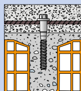
Solaio esistente con caldana
