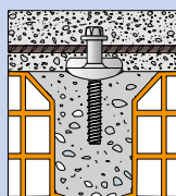
Solaio esistente senza caldana
