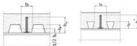
Bac acier avec nervures ouvertes. Bac acier avec nervures rentrantes
